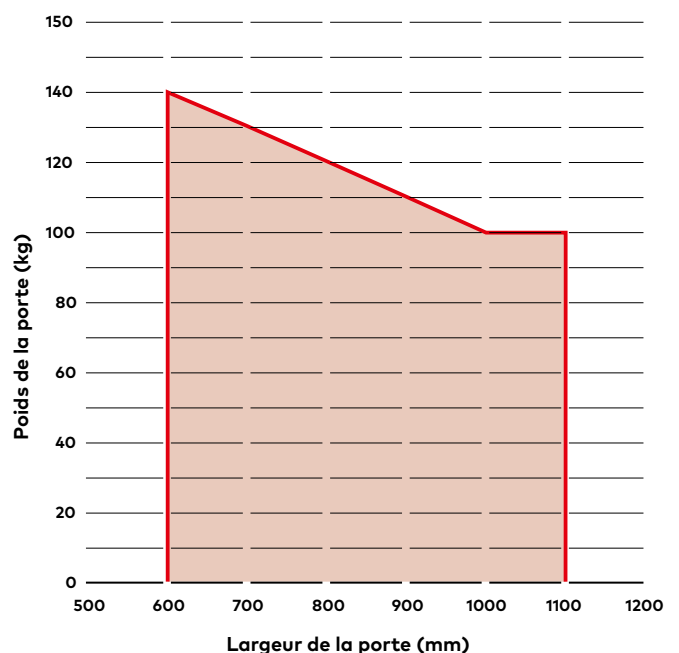
Largeurs et poids de porte maxi. admis
